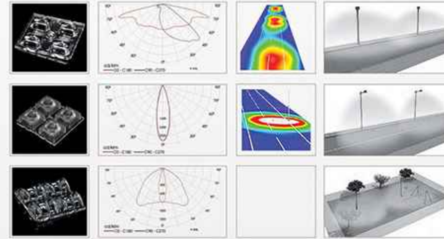
LEDİL C13299 STRADA 2x2 ME
